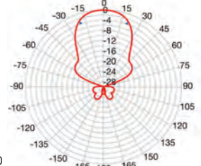
Guadagno (x: frequenza MHz, y: guadagno ISO dBi) e Pattern (@600MHz)
